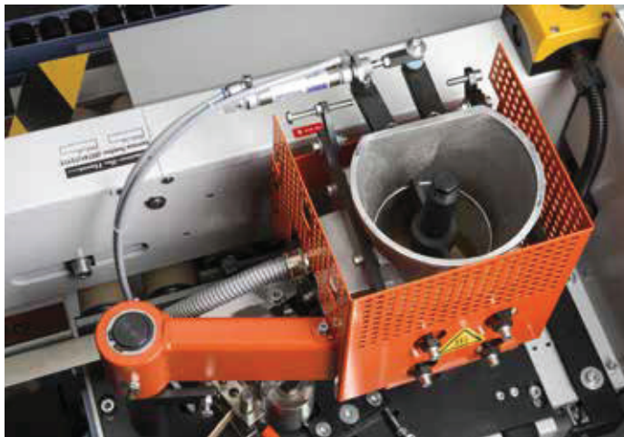
Zelfsluitend bovenliggend lijmbekken.
